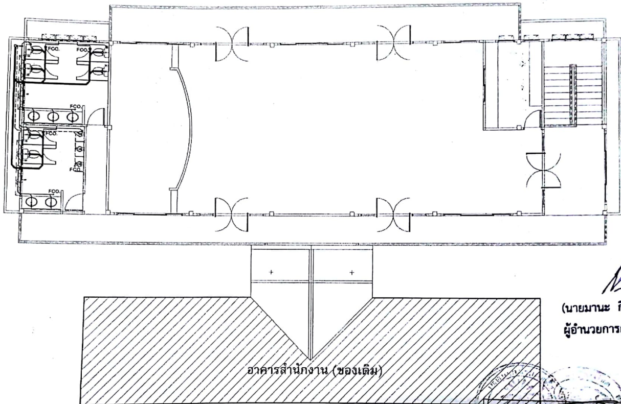
แปลนระบบสุขาภิบาลชั้นที่ 3 มาตราส่วน 1 : 100
