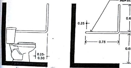
แบบขยายราวจับแบบตัวแอล มาตราส่วน 1 : 25
