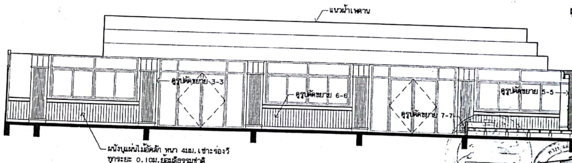
รูปด้านที่ 8 มาตราส่วน 1 : 75
