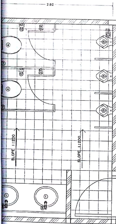
แบบขยายห้องน้ำชาย 3 มาตราส่วน 1 : 25
