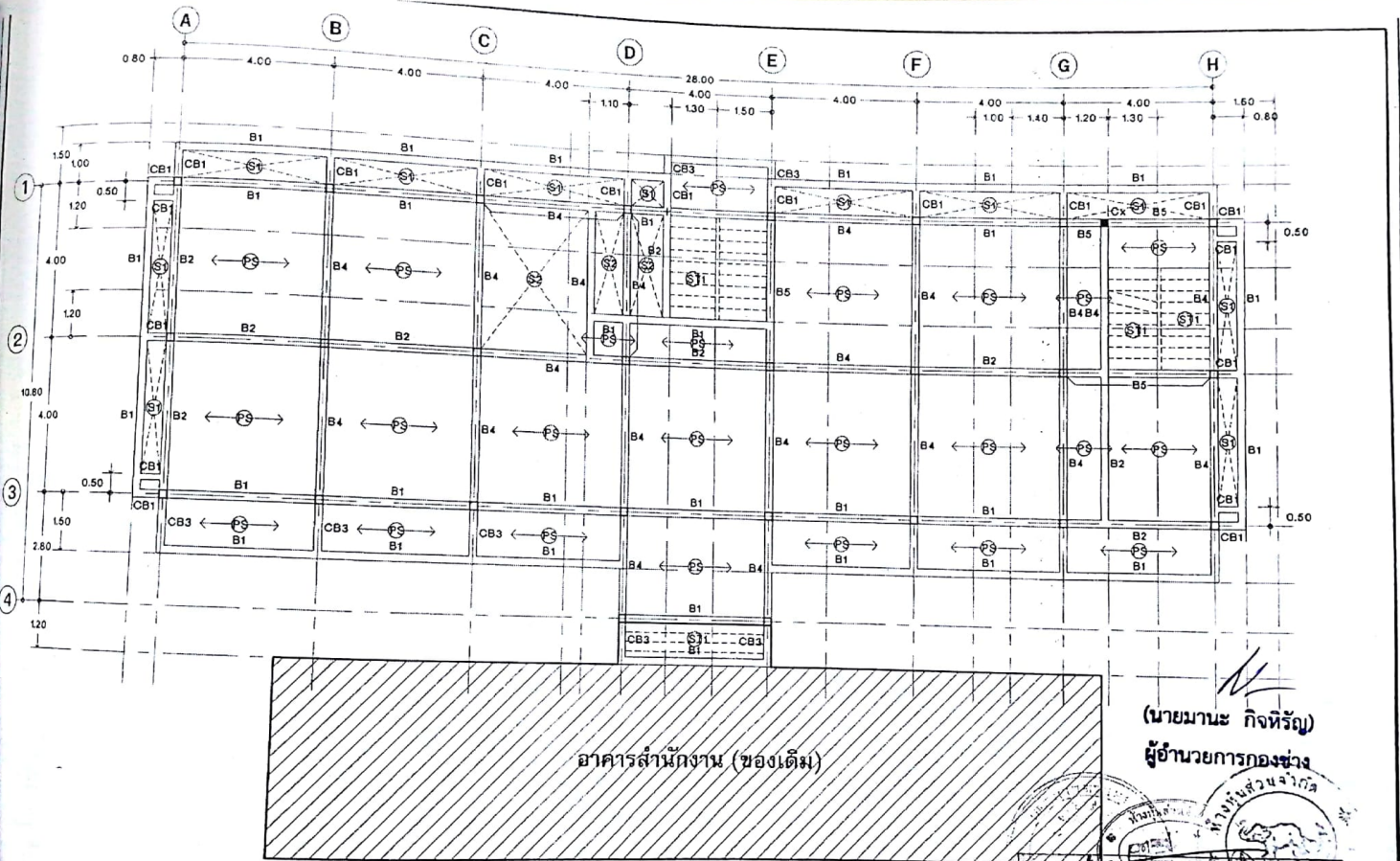
แปลนโครงสร้างชั้นที่ 2 มาตราส่วน 1 : 100
