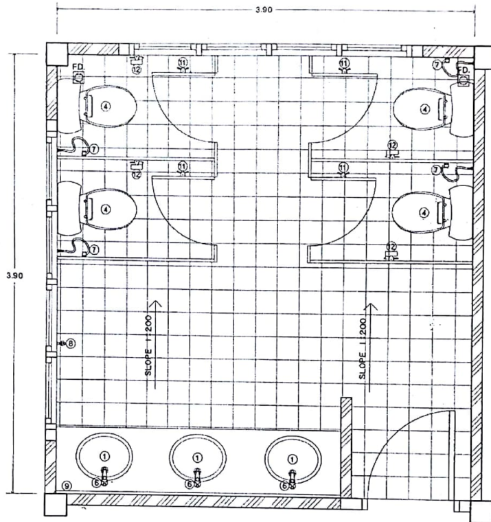
แบบขยายห้องน้ำหญิง 3 มาตราส่วน
