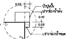
รูปตัดขยาย
