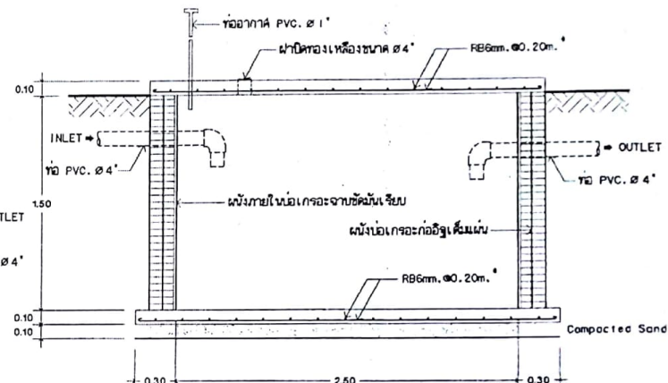
รูปตัดขวาง มาตราส่วน 1 : 25
