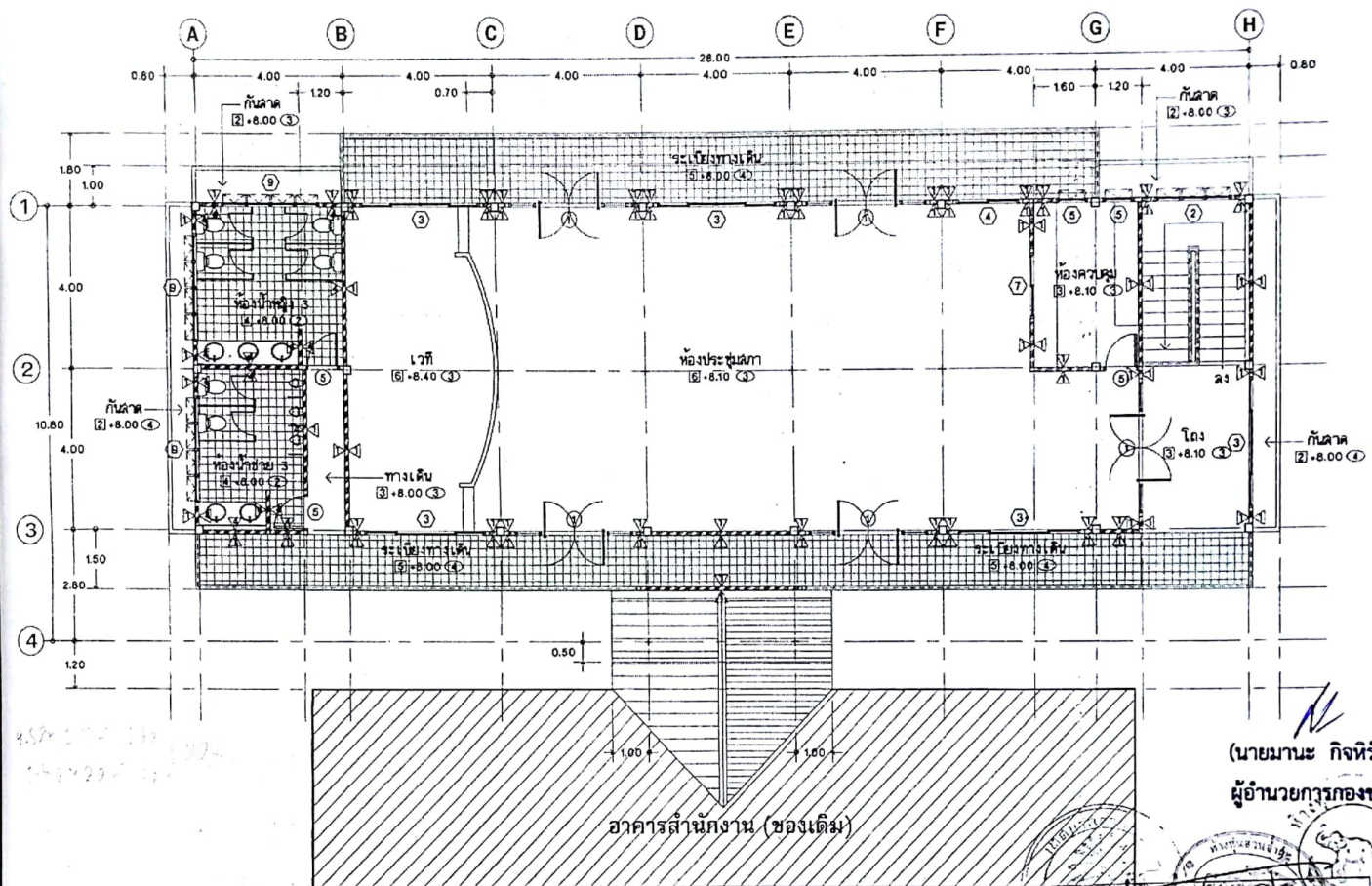
แปลนพื้นที่ 3 มาตราส่วน 1 : 100
