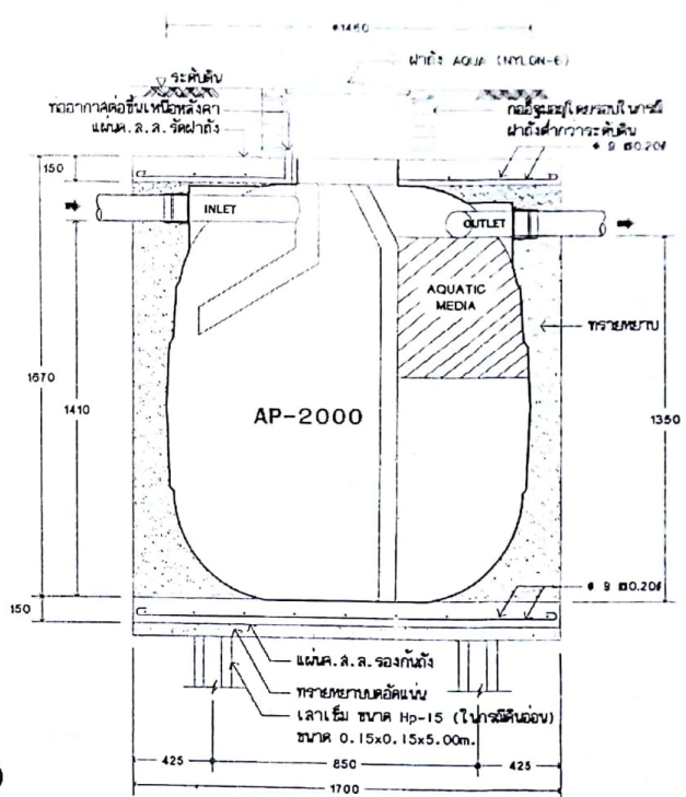
รูปตัดขยายถึงบ้ำบัดน้ำเสีย มาตราส่วน NOT TO SCALE
