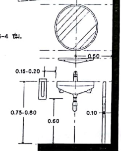
แบบขยายราวจับ, แบบพับเก็บได้ตามแนวดิ่ง มาตราส่วน 1 : 25
