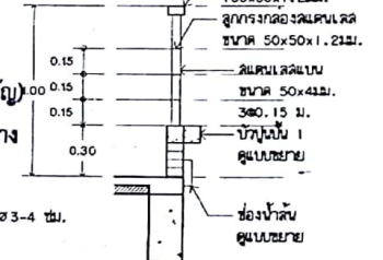
รูปตัดที่ 12-12 มาตราส่วน 1 : 25
