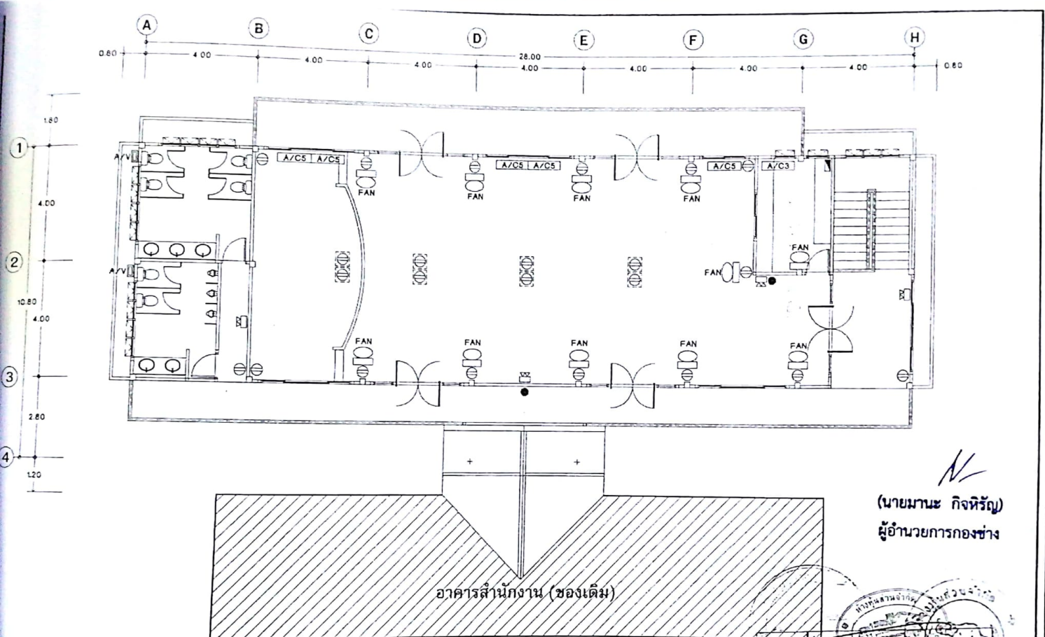
แปลนระบบไฟฟ้ากำลังชั้นที่ ๑ มาตราส่วน 1 : 100
