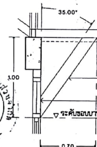
แบบขยายค้ำยันเหล็ก มาตราส่วน 1 : 25
