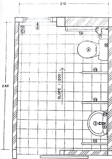
แบบขยายห้องน้ำผู้พิการ มาตราส่วน 1 : 25
