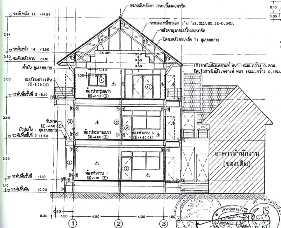
รูปตัดที่ 2-2 มาตราส่วน 1 : 100
