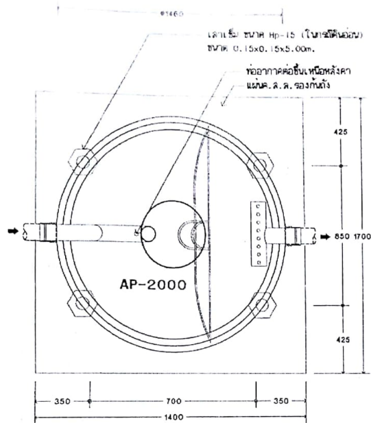
แปลนขยายถึงบ้ำบัดน้ำเสีย มาตราส่วน NOT TO SCALE
