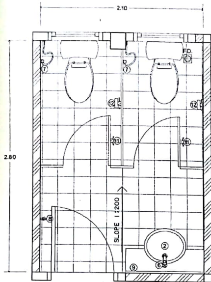
แบบขยายห้องน้ำหญิง 2 มาตราส่วน 1 : 25
