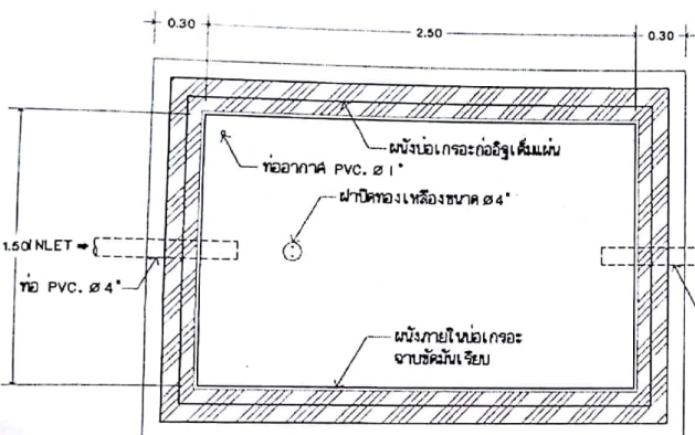
แปลนพื้น มาตราส่วน 1 : 25
